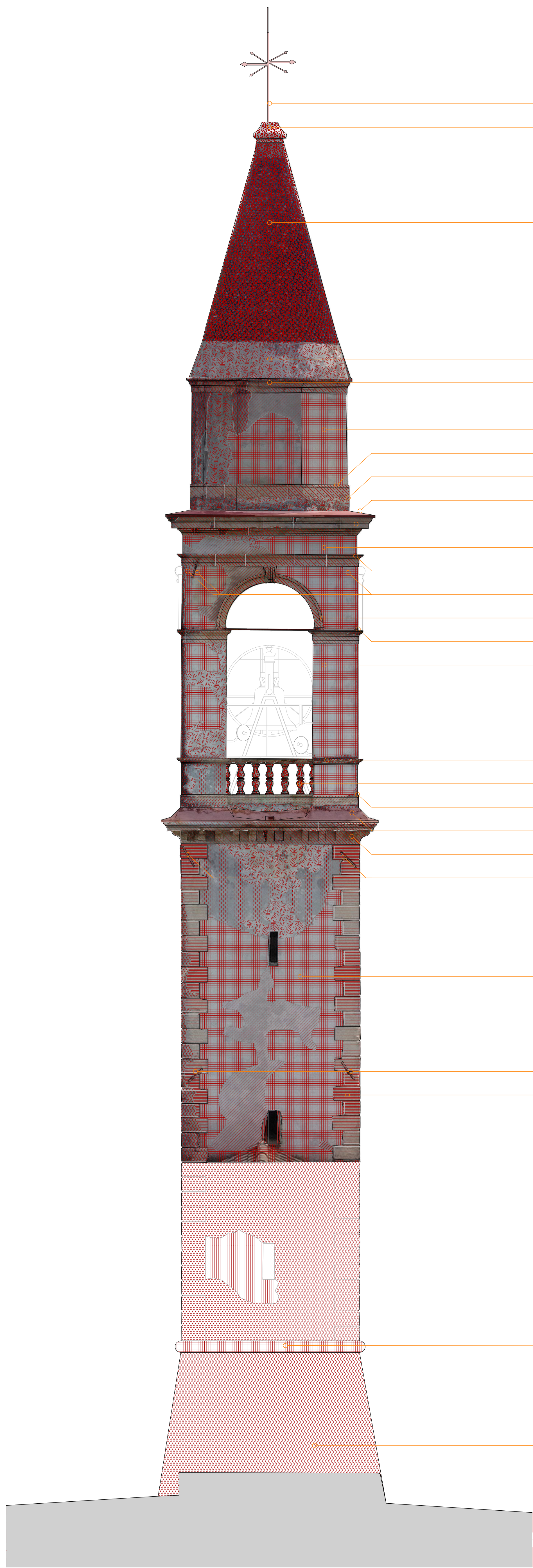
Prospetto Ovest - Rilievo Materico e degradi scala 1.50
