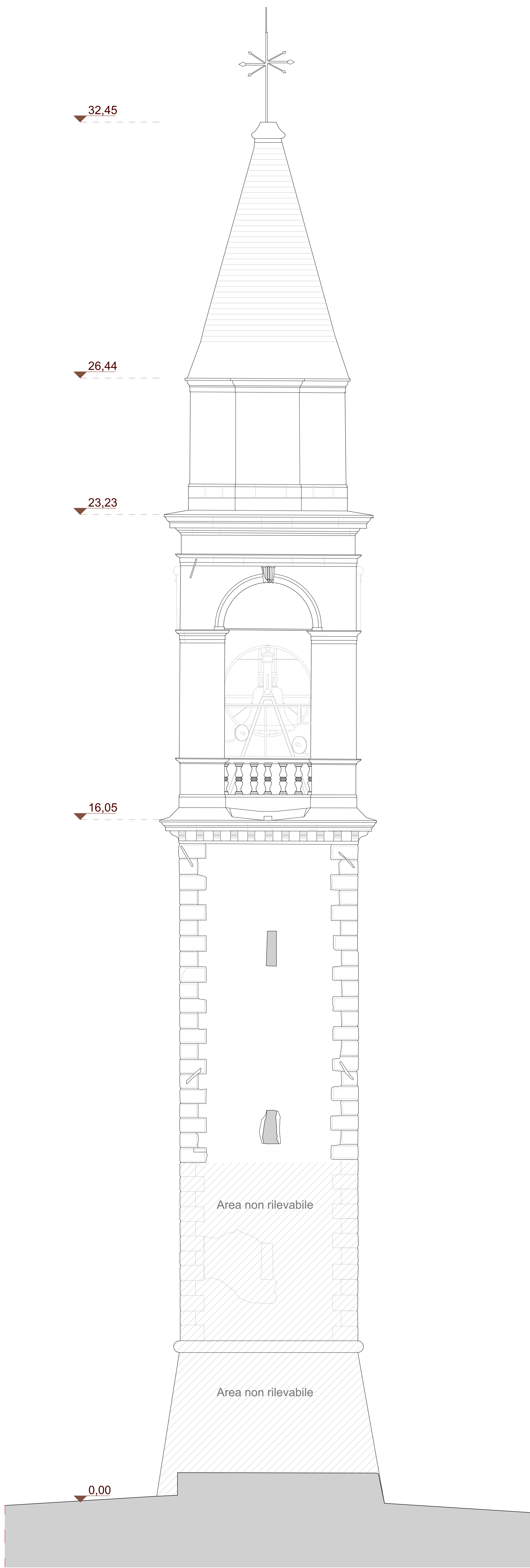
Prospetto Ovest - Rilievo Metrico scala 1.50
