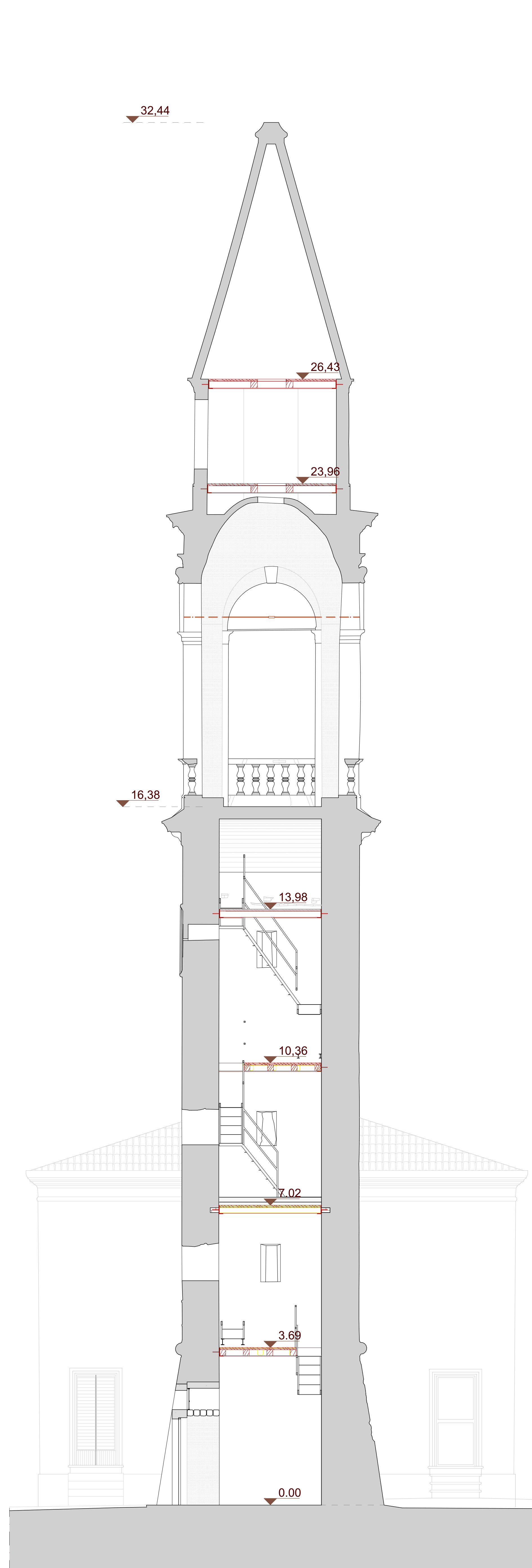
Sezione CC - Comparativa scala 1.50
