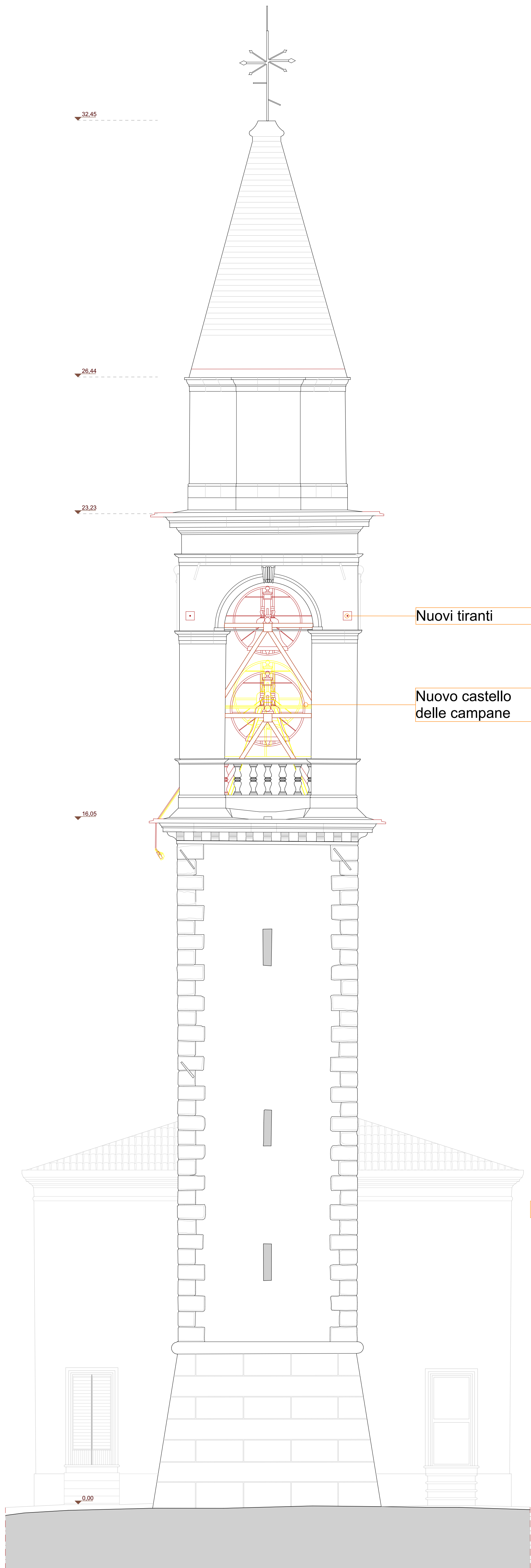
Prospecto Est - Comparativa scala 1.50
