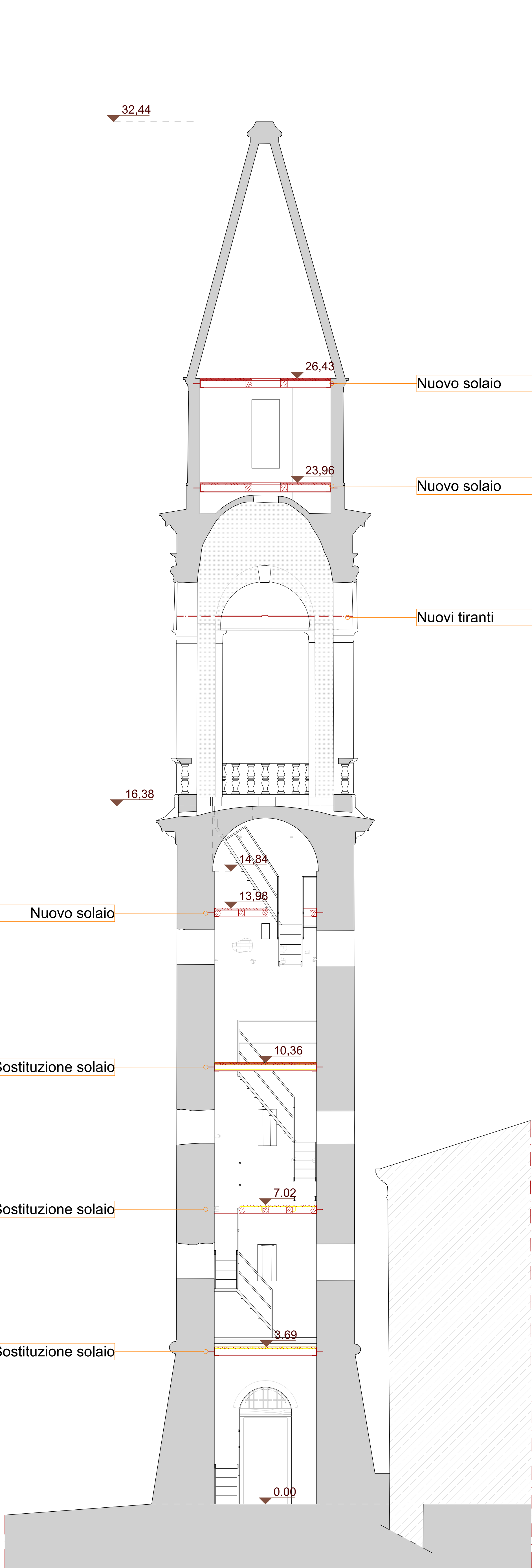
Sezione DD - Comparativa scala 1.50
