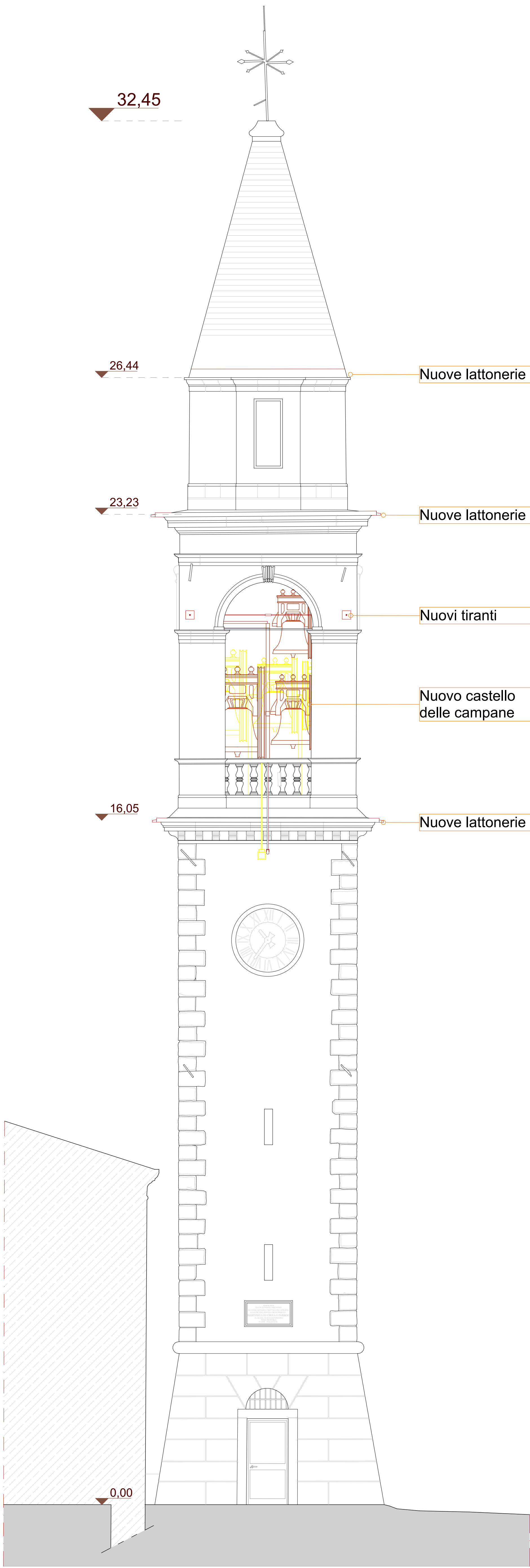
Prospecto Sud - Comparativa scala 1.50
